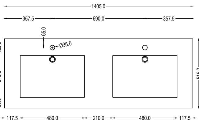
Waschtisch Ausführung HPL stratificato 926 lavabo exécution HPL stratificato 926 lavabo esecuzione HPL stratificato 926
