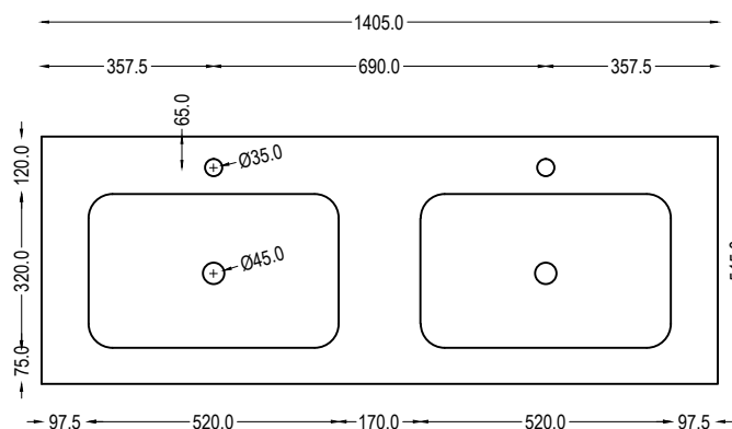
Waschtisch Ausführung Glas 689 + 690 lavabo exécution verre 689 + 690 lavabo esecuzione vetro 689 + 690
