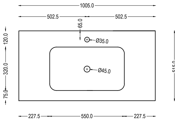
Waschtisch Ausführung Glas 689 + 690 lavabo exécution verre 689 + 690 lavabo esecuzione vetro 689 + 690
