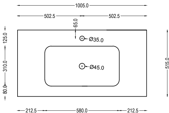
Waschtisch Ausführung Mineralmarmo 486 + 487 lavabo exécution mineralmarmo 486 + 487 lavabo esecuzione mineralmarmo 486 + 487
