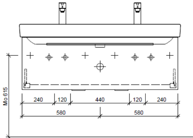
Typ PRO S-RANA 120e
