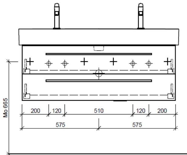
Typ VAL-RANA 120f
