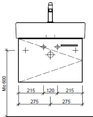
Typ ME-TORO 60a
