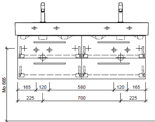
Typ VAL-RANA 120I
