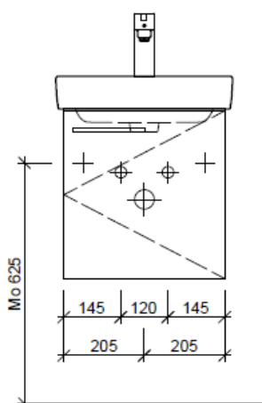
Typ PRO S-TORO 45b
