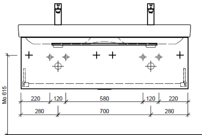
Typ PRO S-RANA 130a
