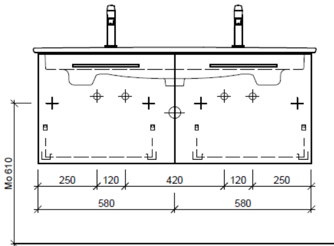
Typ VC-TORO 120c
