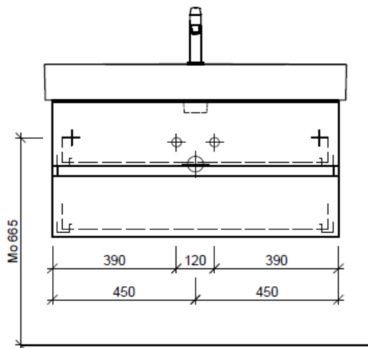
Typ VAL-TORO 95c GLH
