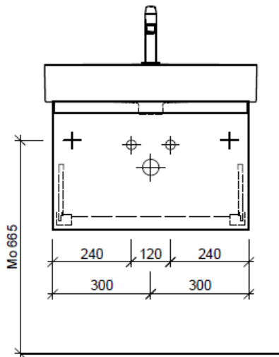
Typ VAL-GATTO 65a
