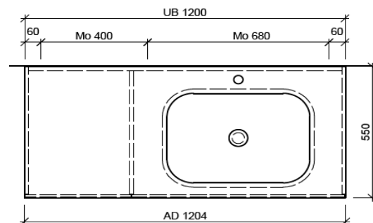
Becken: Corner II, 619 Mineralstoff weiss Grösse: 500 x 340 x 125 mm (ohne Überlauf)
