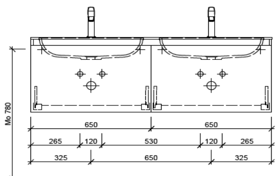
Becken: Wave II, 5337 Mineralstoff weiss Grösse: 535 x 375 x 100 mm (ohne Überlauf)
