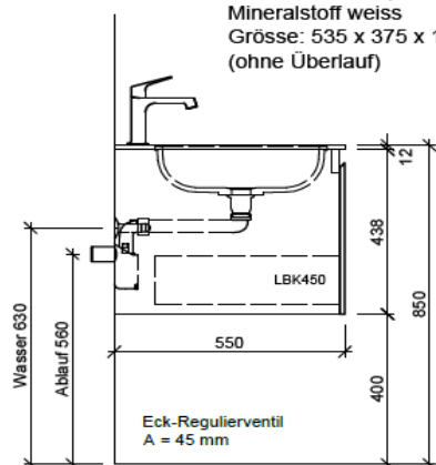
team 855 107 Raumspär-Sifon Geberit 5/4" x 40 mm Kunststoff weiss
