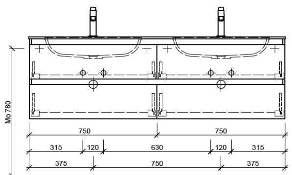
Becken: Wave II, 5337 Mineralstoff weiss Grösse: 535 x 375 x 100 mm (ohne Überlauf)
