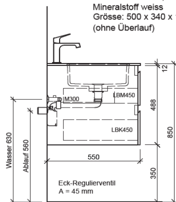
team 855 107 Raumspär-Sifon Geberit 5/4" x 40 mm Kunststoff weiss
