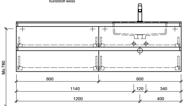
team 855 107 Raumspär-Sifon Geberit 5/4" x 40 mm Kunststoff weiss
