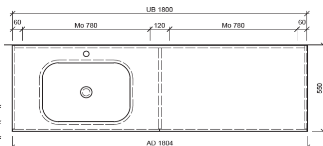
Becken: Corner II, 619 Mineralstoff weiss Grösse: 500 x 340 x 125 mm (ohne Überlauf)
