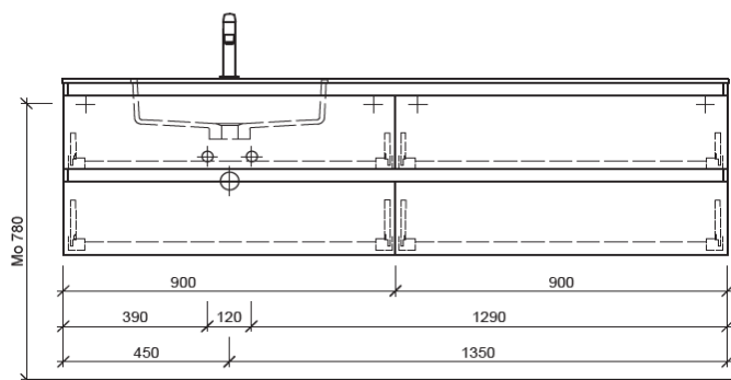
team 855 107 Raumsparsifon Geberit 5/4" x 40 mm Kunststoff weiss
