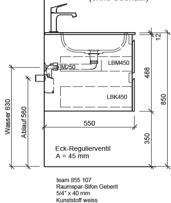
Becken: Wave II, 5337 Mineralstoff weiss Grösse: 535 x 375 x 100 mm (ohne Überlauf)
