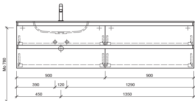
Becken: Wave II, 5337 Mineralstoff weiss Grösse: 535 x 375 x 100 mm (ohne Überlauf)
