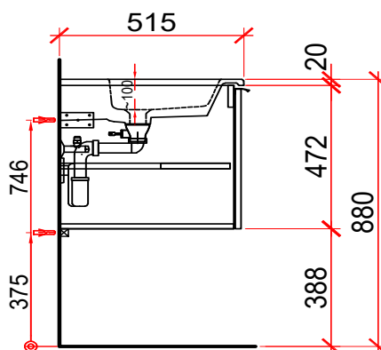
Decoupe pour siphon reduit Ausschnitt für Raumspar-siphon
