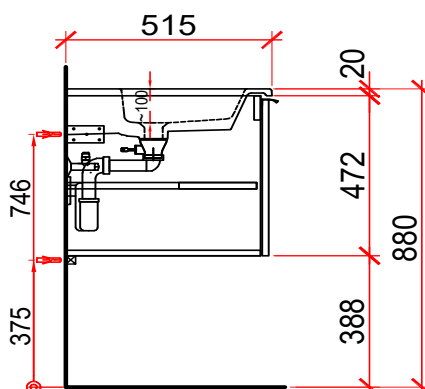
Decoupe pour siphon réduit Ausschnitt für Raumspar-siphon
