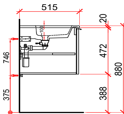
Decoupe pour siphon réduit Ausschnitt für Raumspar-siphon
