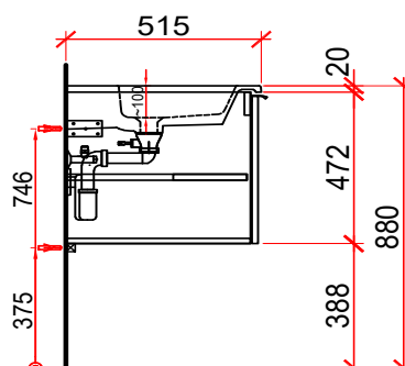
Decoupe pour siphon réduit Ausschnitt für Raumspar-siphon
