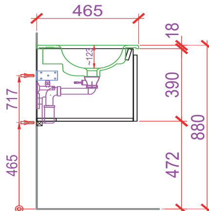
Decoupe pour siphon réduit Ausschnitt für Raumspar-siphon
