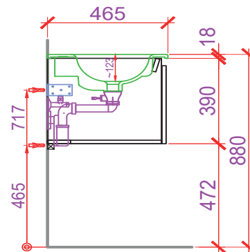
Decoupe pour siphon réduit Ausschnitt für Raumspar-siphon
