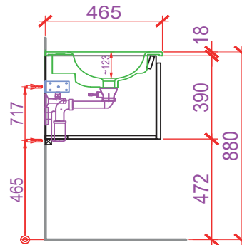
Decoupe pour siphon réduit Ausschnitt für Raumspar-siphon
