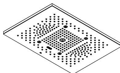
Deckenmodul mit Lichtkontroller und LED Ceiling module with light controller and LED
