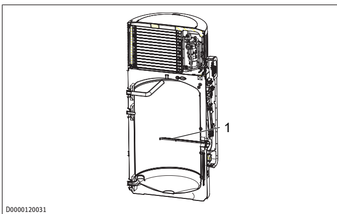
1 elektrische Not-/Zusatzheizung
