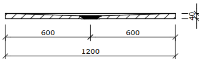
Schnitt A-A (1 : 15)
