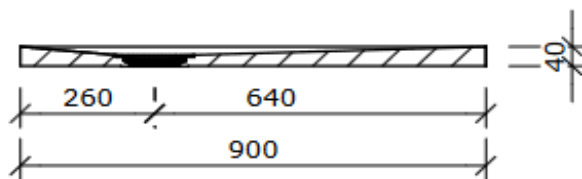
Schnitt A-A (1 : 15)
