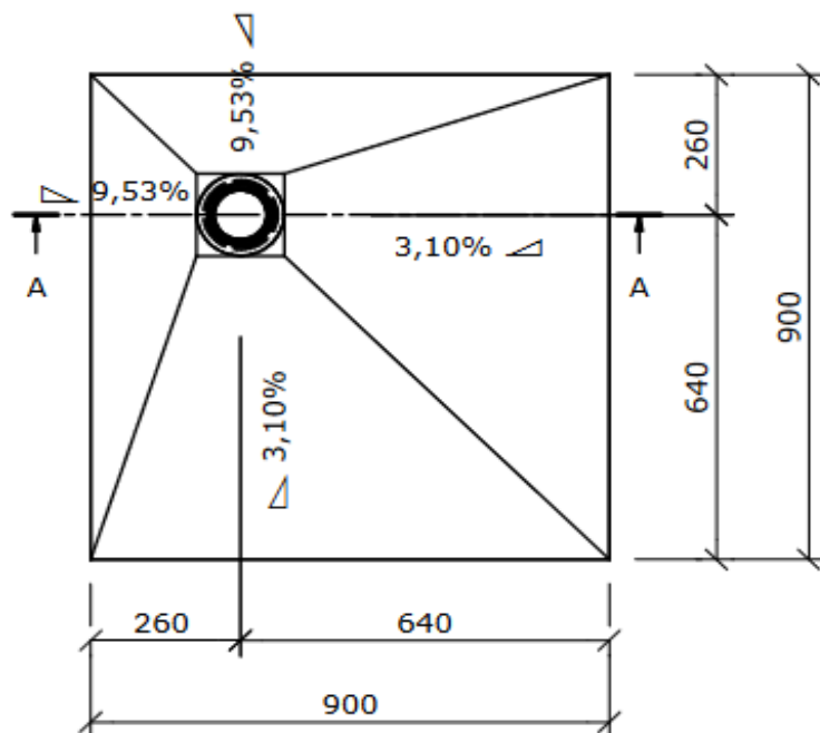
Draufsicht ( 1 : 15 )
