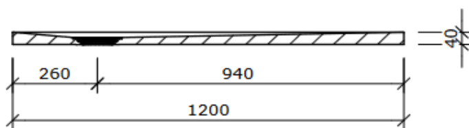
Schnitt A-A (1 : 15)
