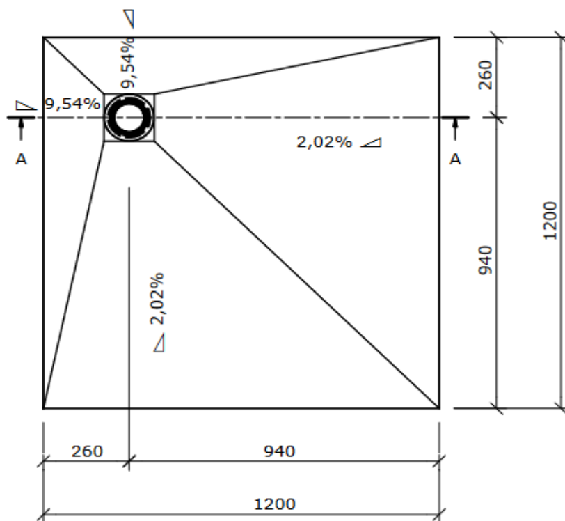
Draufsicht ( 1 : 15 )
