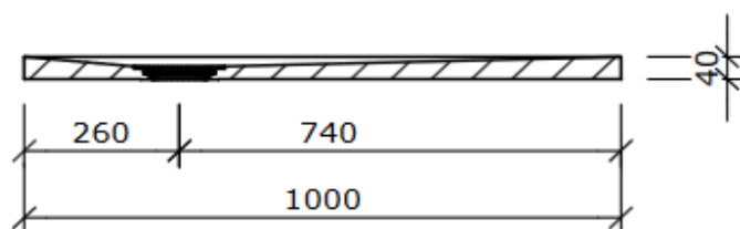
Schnitt A-A ( 1 : 15 )
