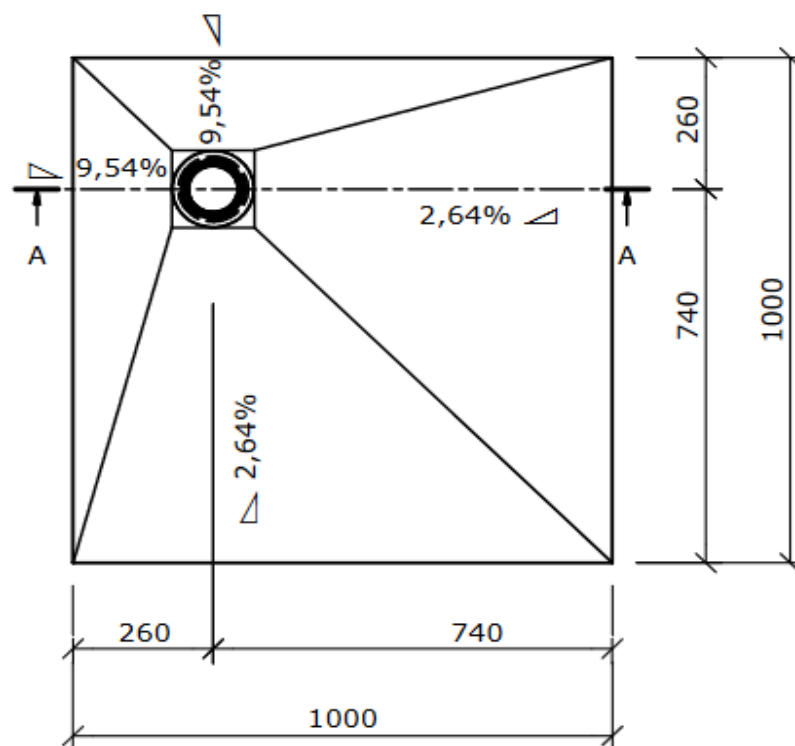
Draufsicht ( 1 : 15 )
