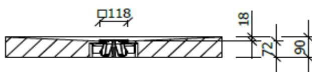
Schnitt A-A (1 : 15)
