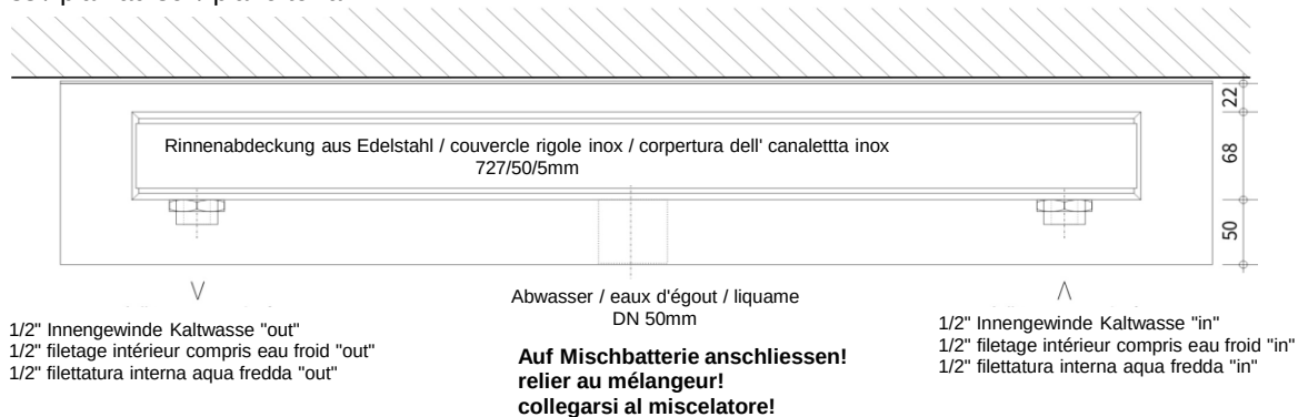
Grundriss / plan au sol / piano terra
