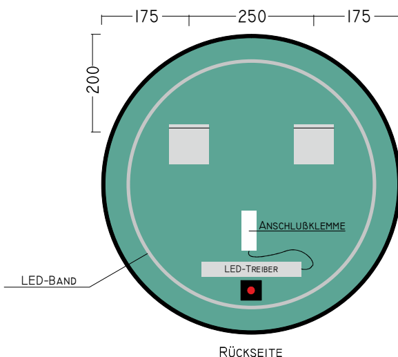
RÜCKANSICHT
