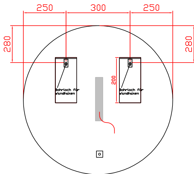
Rückseite
