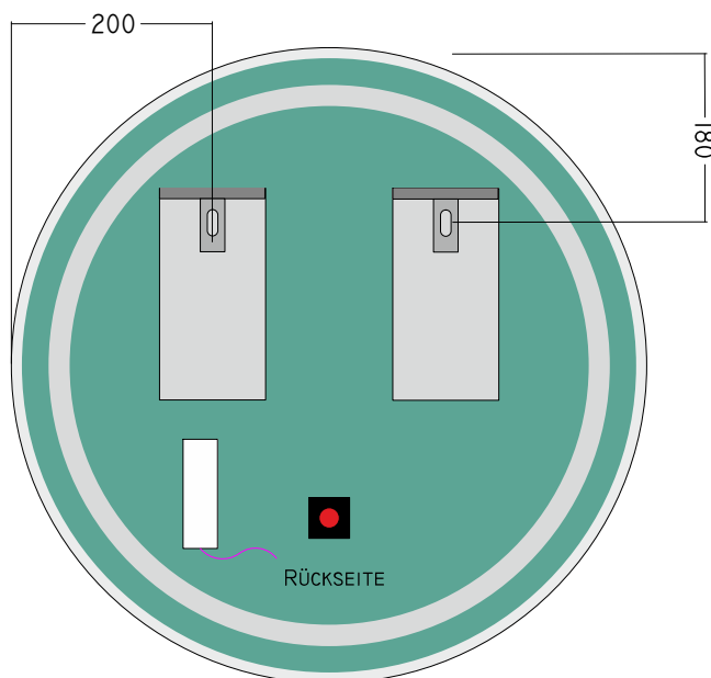
RÜCKANSICHT
