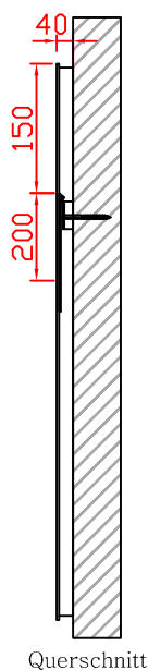
Querschnitt
