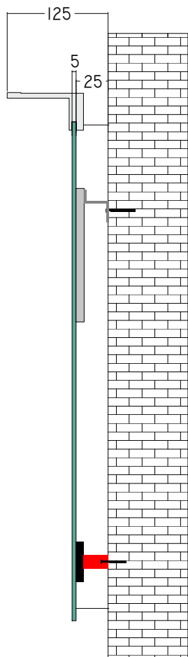
SEITENANSICHT
