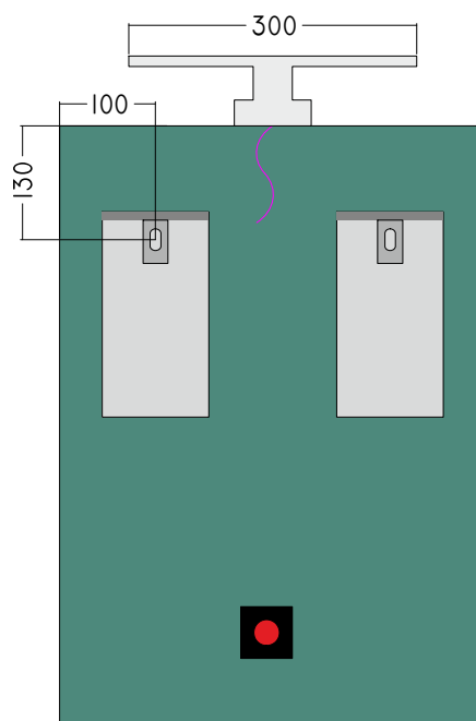
RÜCKANSICHT
