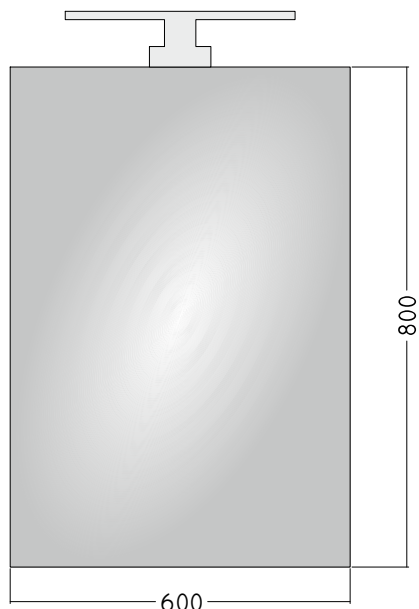
FRONTANSICHT
