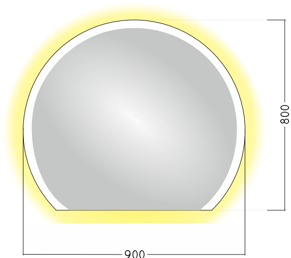
FRONTANSICHT
