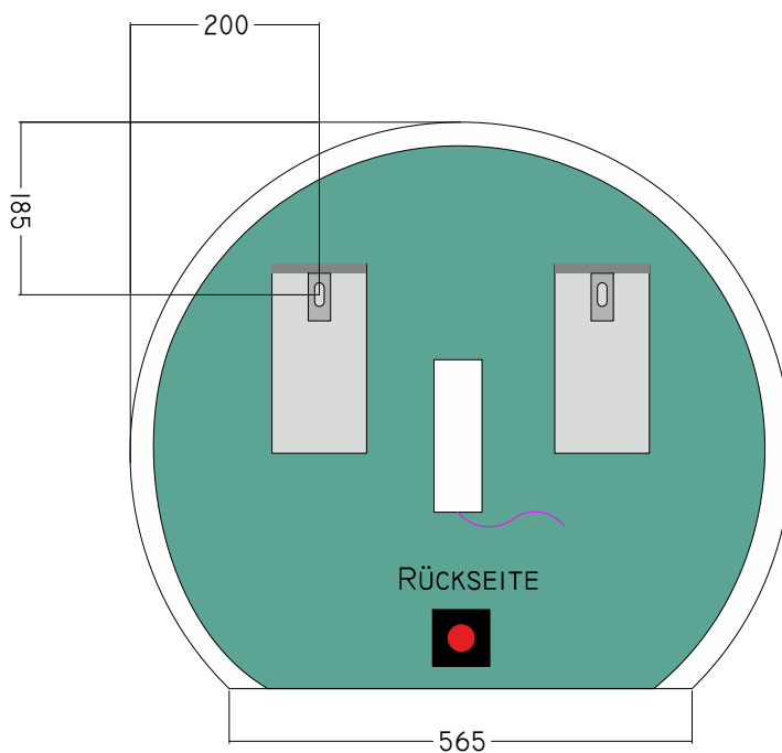
RÜCKANSICHT
