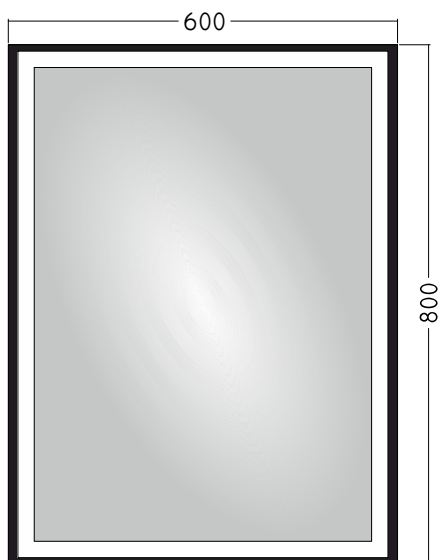
FRONTANSICHT
