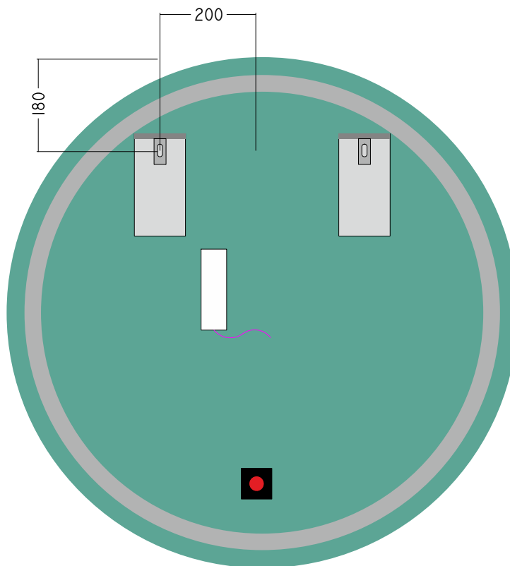
RÜCKANSICHT
