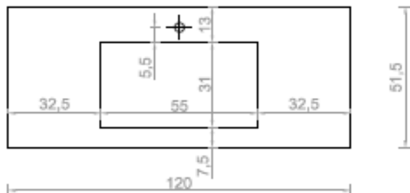
DRAUFSICHT
