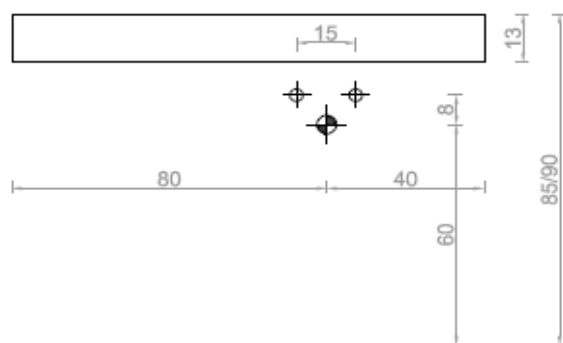
DRAUFSICHT
