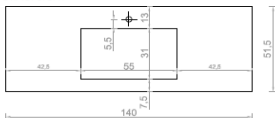
DRAUFSICHT
