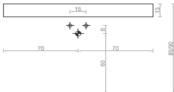
DRAUFSICHT
