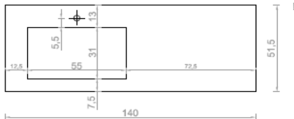
DRAUFSICHT
