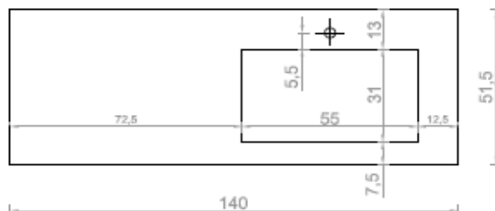
DRAUFSICHT
