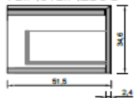
SCHNITTANSICHT FEINSTEINZEUG
