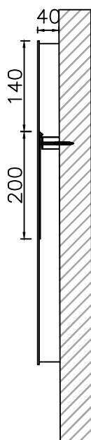
Querschnitt
