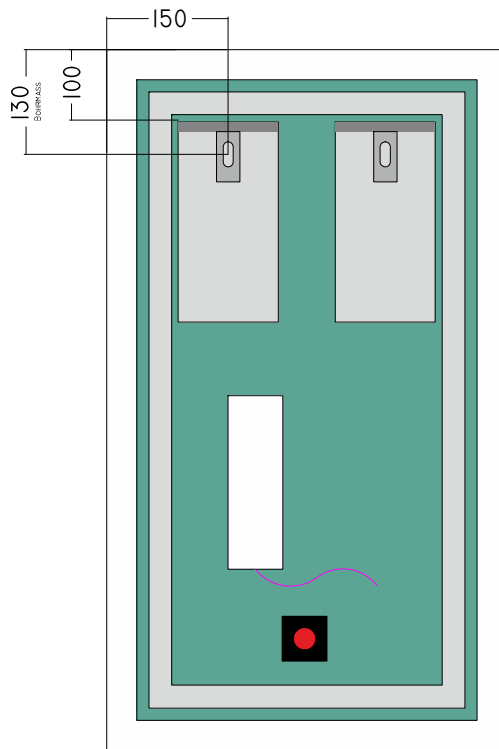
RÜCKANSICHT
