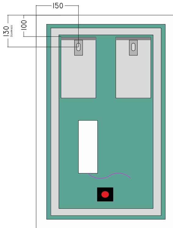
RÜCKANSICHT
