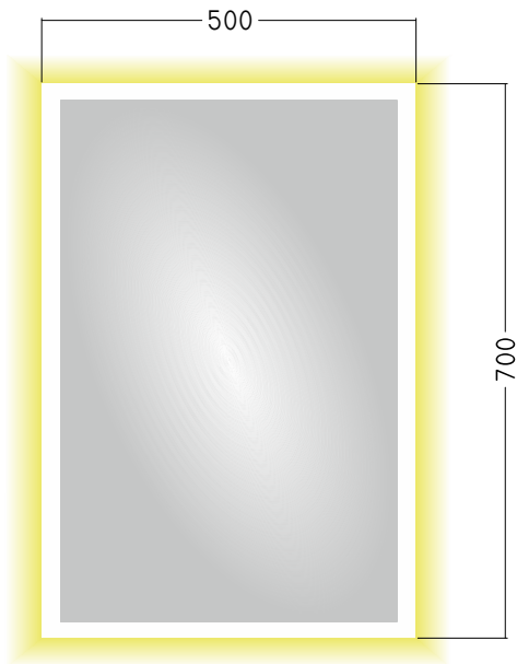
FRONTANSICHT
