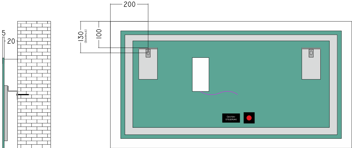
FRONTANSICHT
