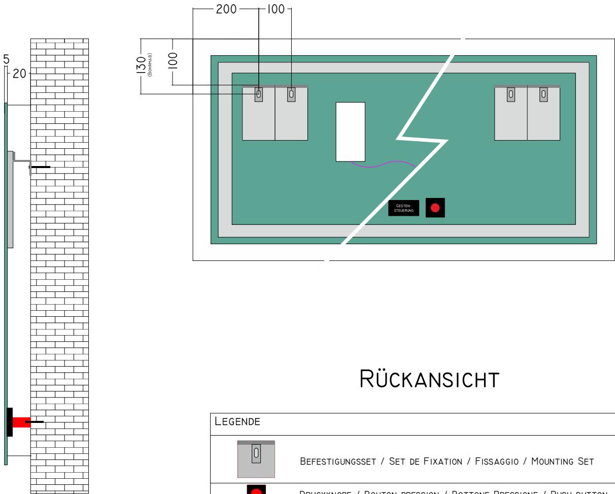
FRONTANSICHT
